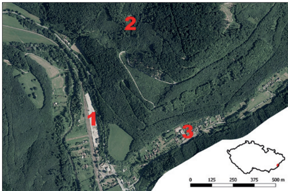
Obr. 1. Vlárský průmysk se značenými lokalitami výzkumu. 1- expediční sklad dřeva ve stanici Vlárský průmysk, 2 – lom pod PP Okrouhlá, 3 – osada Sidonie. Zdroj: Geoportál ČÚŽK, dostupné na http://geoportal.cuzk.cz .
