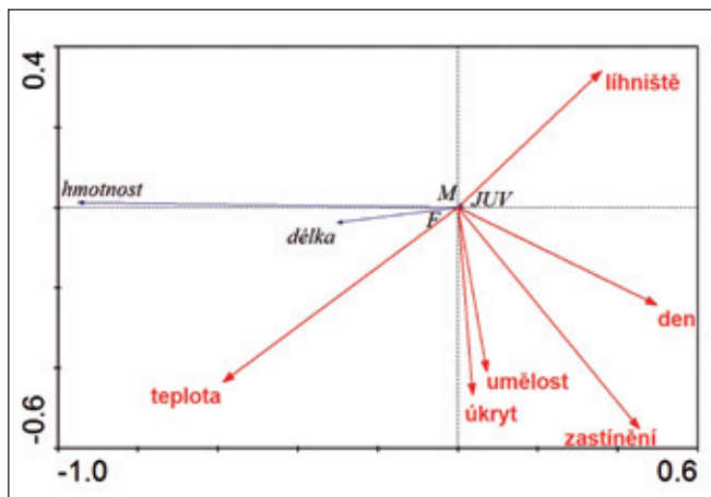
Obr. 9. Ordinační diagram RDA analýzy. Druhov data jsou v dvourozměrném prostoru umístěny ve vztahu k jednotlivým faktorům prostředí. Ze všech faktorů prostředí byly statisticky významné: teplota – LambdaA = 0,14, p = 0,002, F = 12,15; den v roce – LambdaA = 0,17, p = 0,002, F = 17,97; zastínění vegetací – LambdaA = 0,08, p = 0,004, F = 8,93 Fig. 9. Ordination diagram of RDA analysis. Species data are situated in 2D space in their relation to each environmental factor. Statistically important were following factors: temperature (teplota) – LambdaA = 0,14, p = 0,002, F = 12,15; day in a year (den v roce) – LambdaA = 0,17, p = 0,002, F = 17,97; vegetation cover (zastínění vegetací) – LambdaA = 0,08, p = 0,004, F = 8,93.
